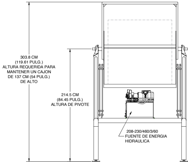
VISTA LATERAL
