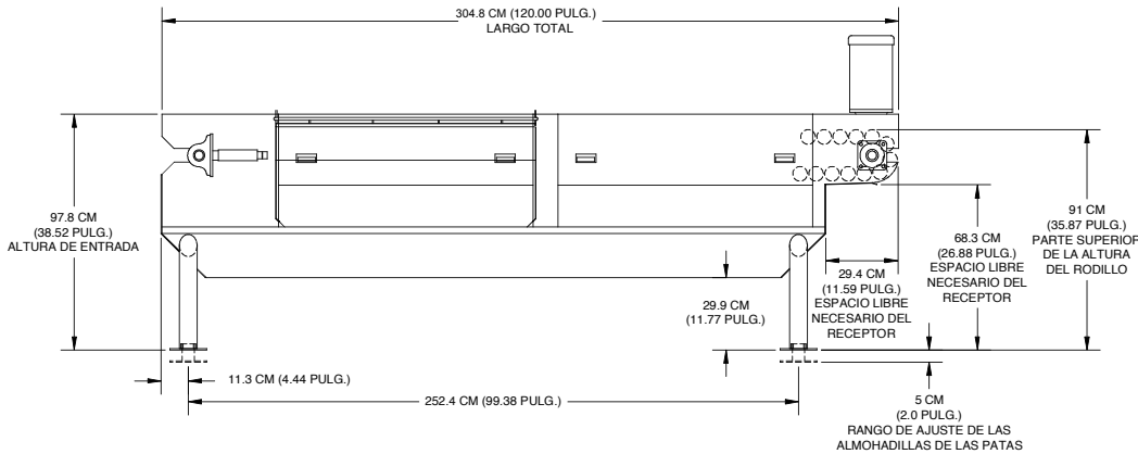
VISTA LATERAL
